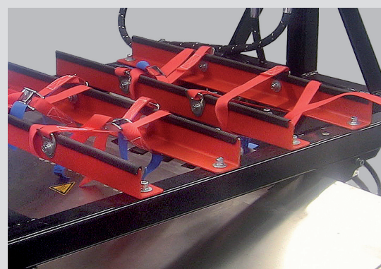
Gasflaschenhalterung auf dem Gerät (Option)
